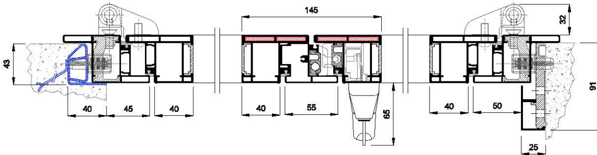
Sezione orizzontale 2 ante
