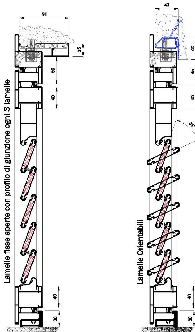
Sezione verticale
